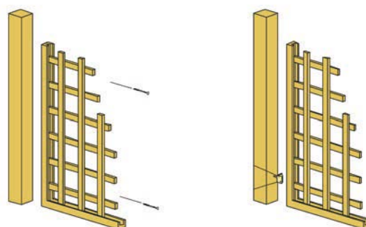
Fissaggio mediante viti mordenti Cod. 21070
